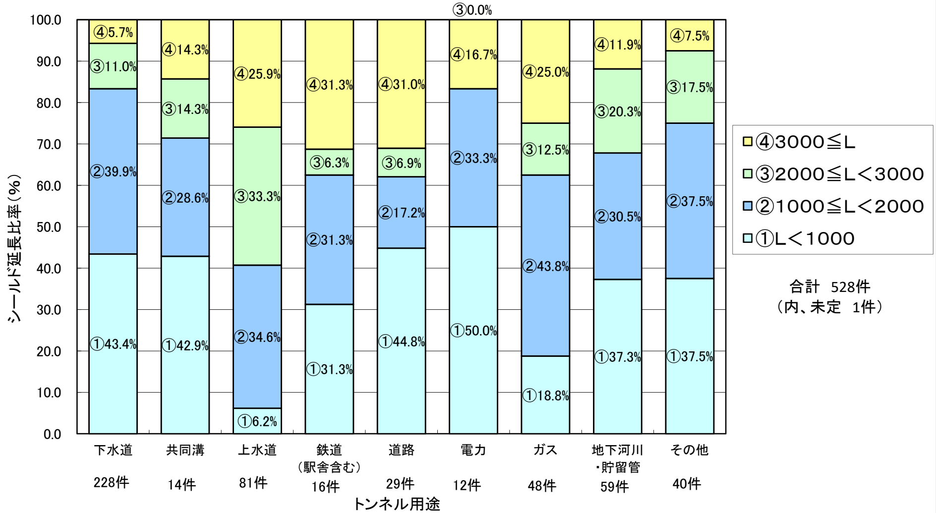
トンネル用途別シールド延長比率('09~'18年度) ※工事件数は契約年度ごとに集計
