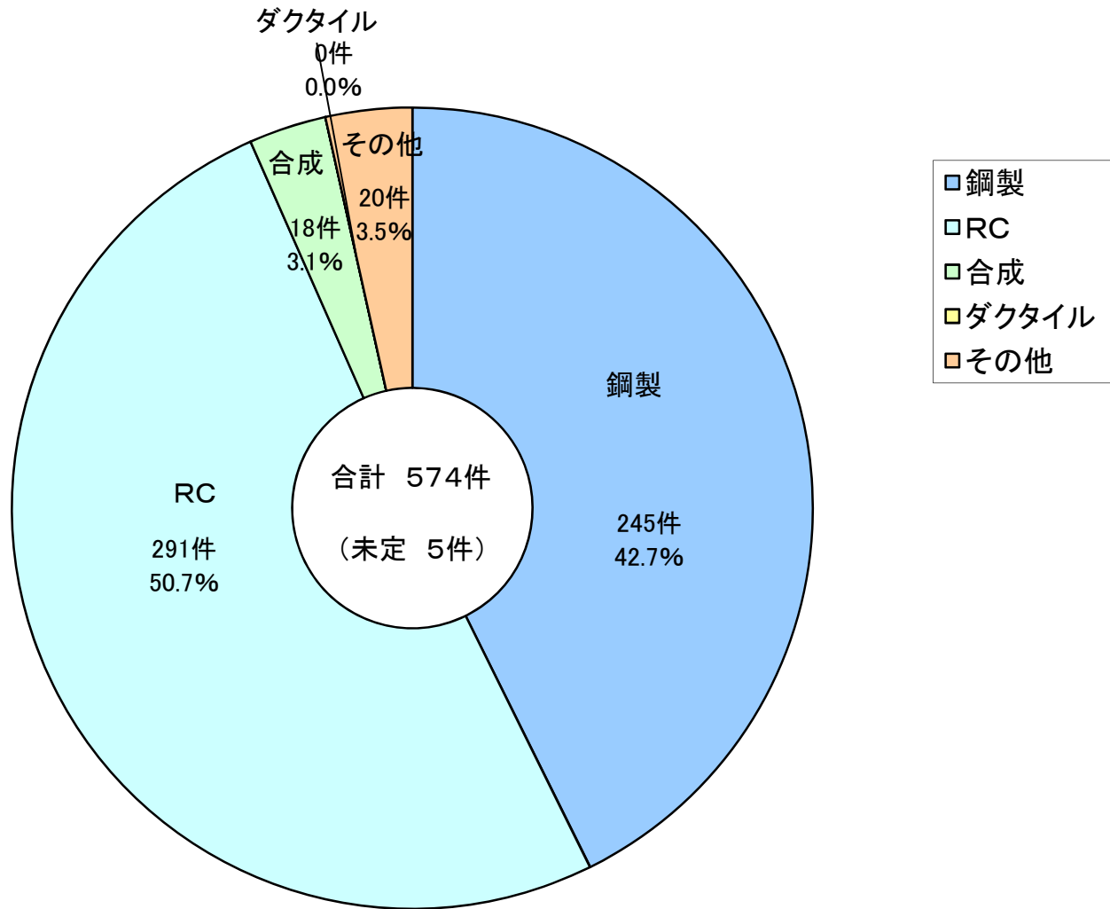
セグメント種別工事件数(2007～2016年度)
