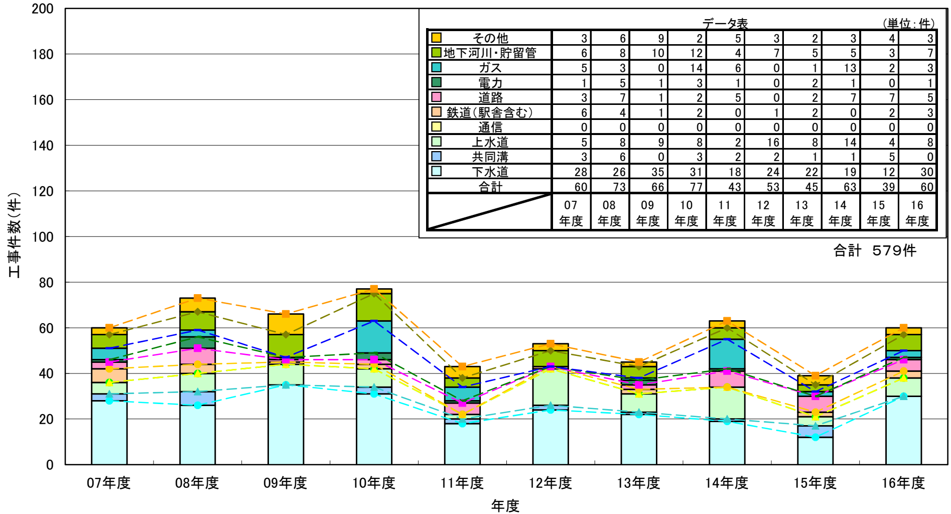
トンネル用途別工事件数(年度別 2007～2016年度)
