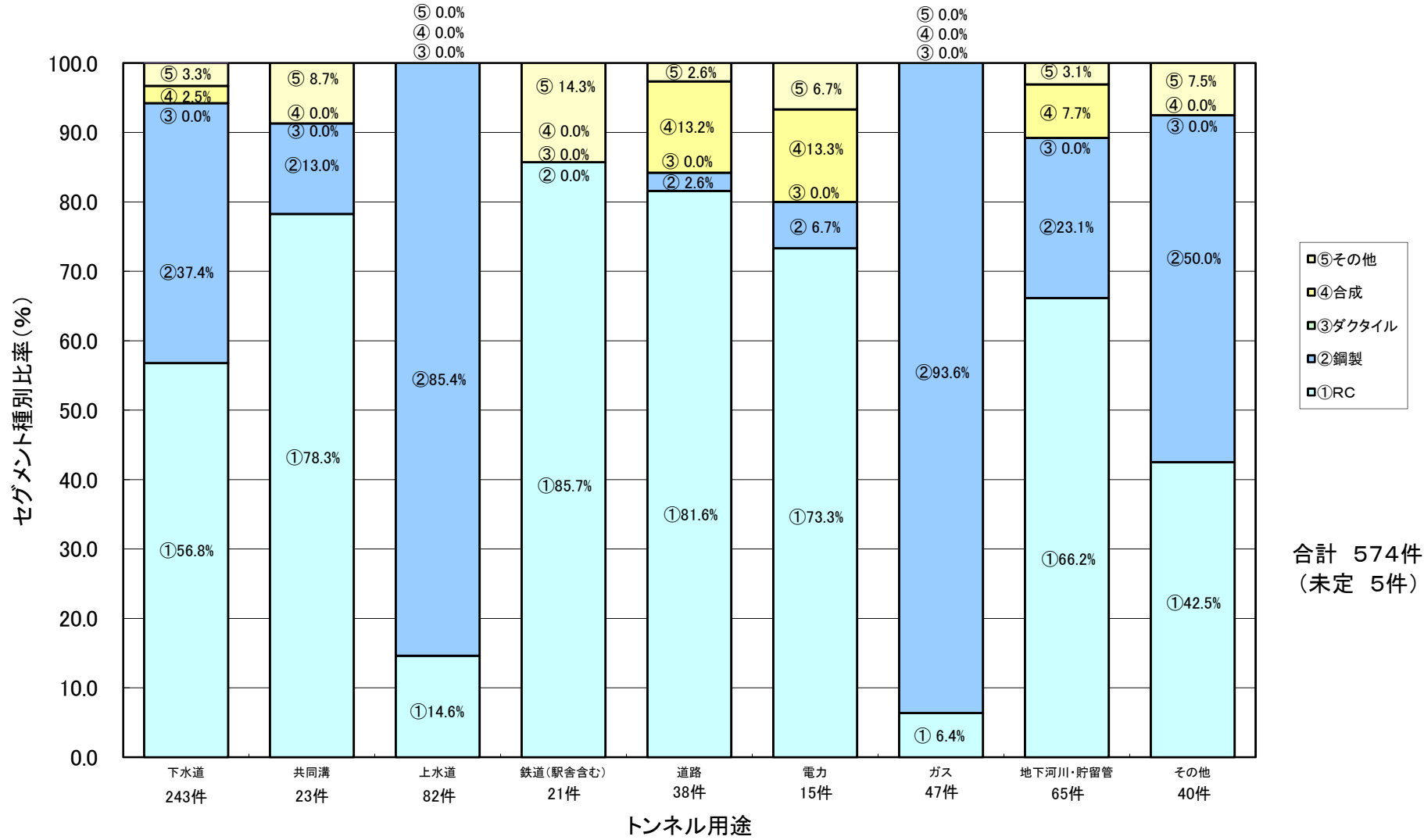
トンネル用途別セグメント種別比率(2007~2016年度)
