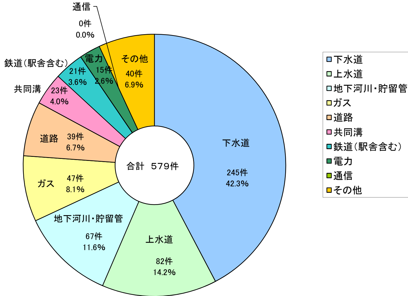
トンネル用途別工事件数(2007~2016年度)
