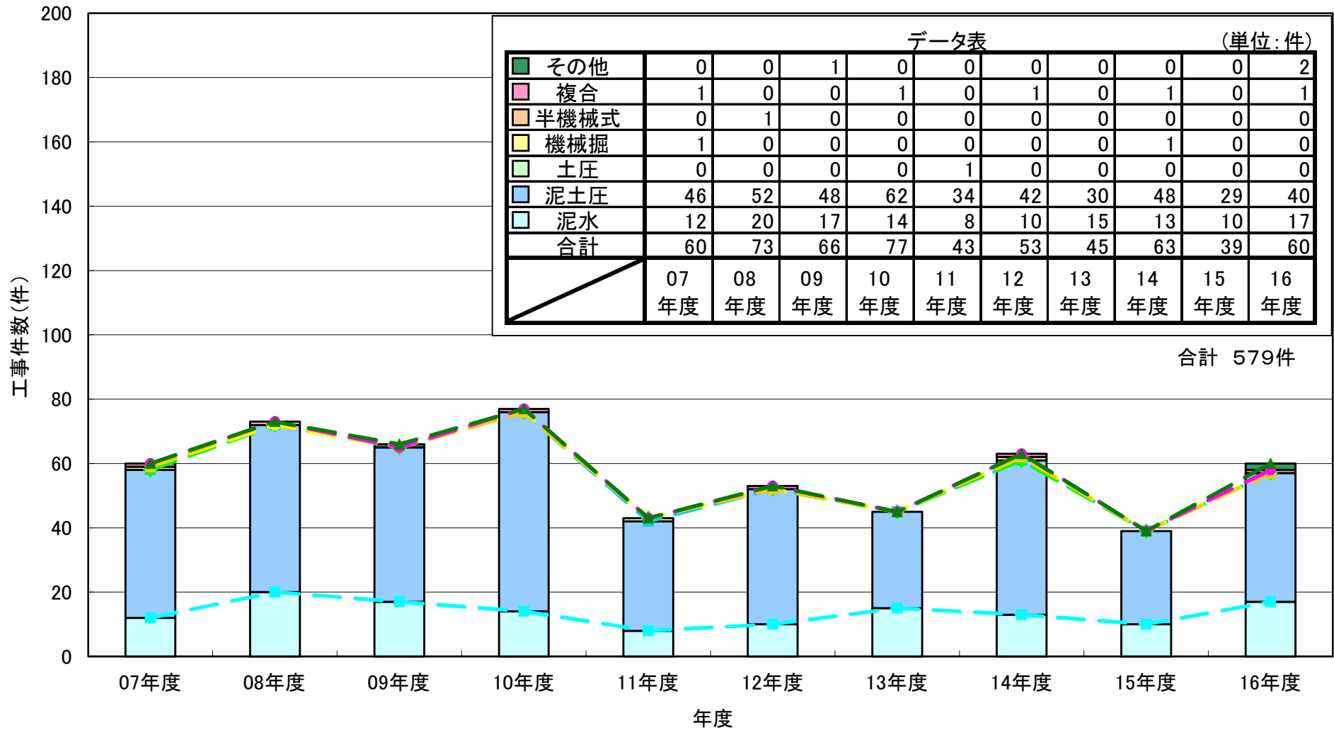
シールド機種別工事件数(年度別 2007～2016年度)
