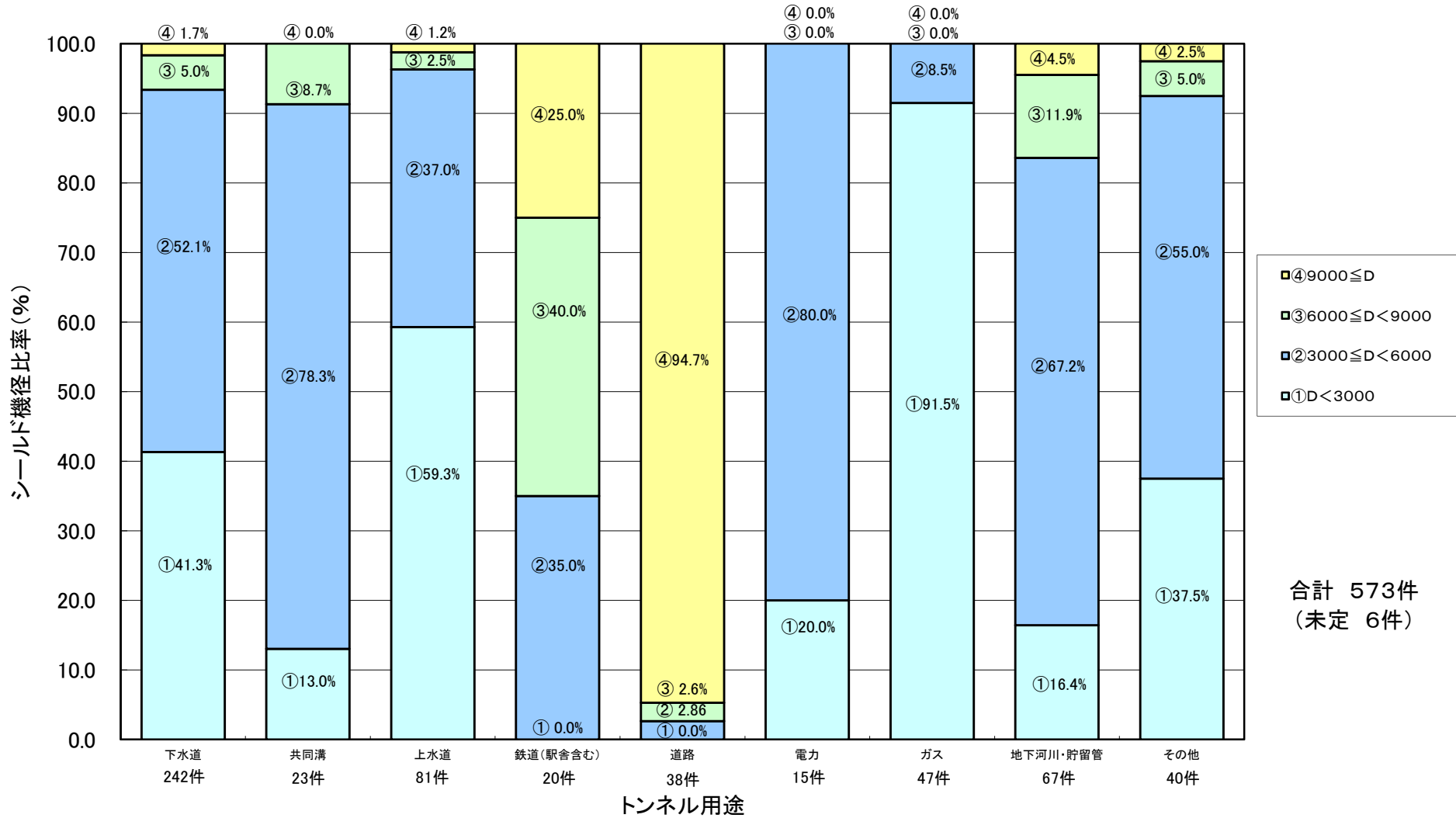
トンネル用途別シールド機径比率(2007~2016年度)
